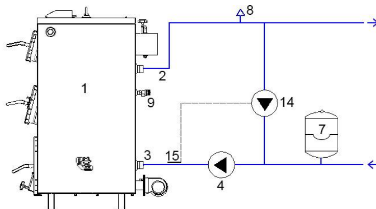
Рис.6 Схема обв'язки котла з бойлером (рекомендована)
